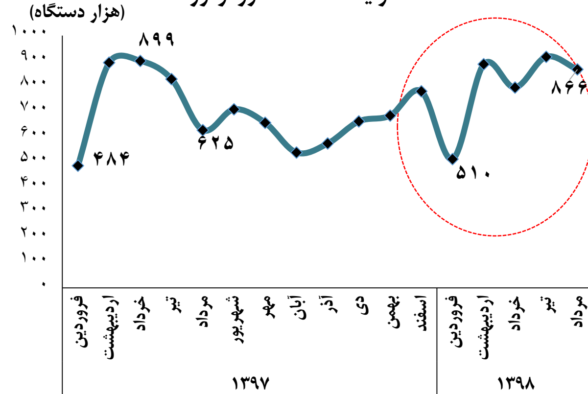
تولید ماهانه الکتروموتور
