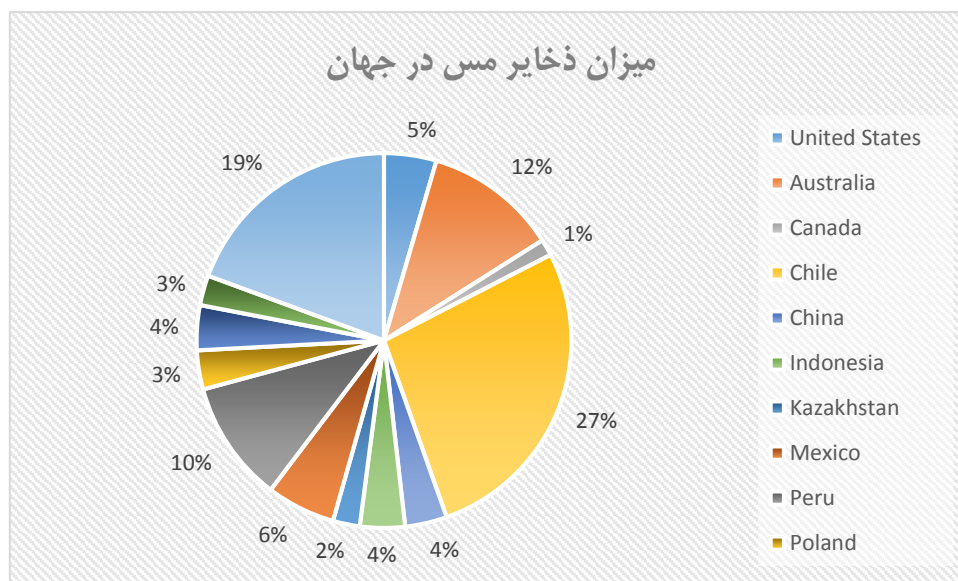
شکل شماره (۳): میزان ذخایر کشورهای تولیدکننده مس (منبع: گزارش سال ۲۰۱۷ سازمان زمین‌شناسی ایالات متحده آمریکا)
