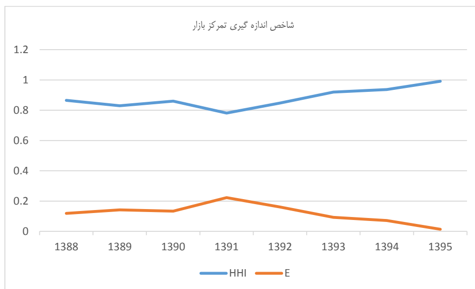
شکل شماره (۸): شاخص اندازه‌گیری تمرکز بازار مس
