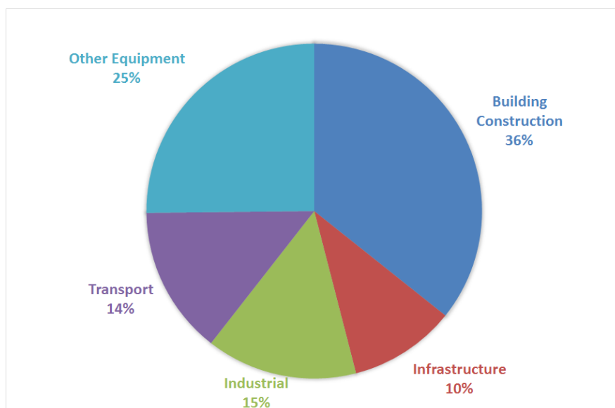
شکل شماره (۶): میزان مصرف مس بر اساس فعالیت (منبع: ICA, ۲۰۱۵, IWCC)
