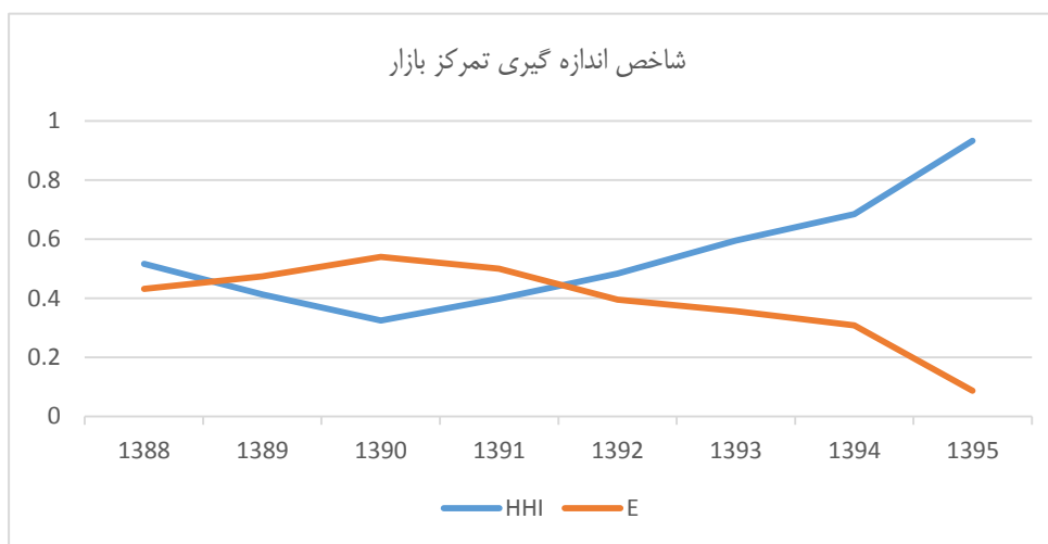
شکل شماره (۱۲): شاخص اندازه‌گیری تمرکز بازار آلومینیوم
