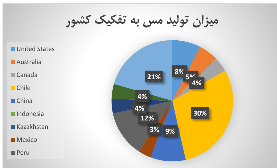
شکل شماره (۴): میزان تولید سال ۲۰۱۶ مس جهانی به تفکیک کشور (منبع: گزارش سال ۲۰۱۷ سازمان زمین‌شناسی ایالات متحده آمریکا)
