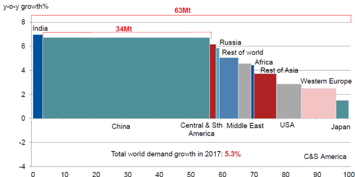
شکل شماره (۱۰): میزان مصرف سال ۲۰۱۷ آلومینیوم جهانی به تفکیک منطقه (منبع: گزارش سال ۲۰۱۷ CRU Aluminium Market OutlookSource)
