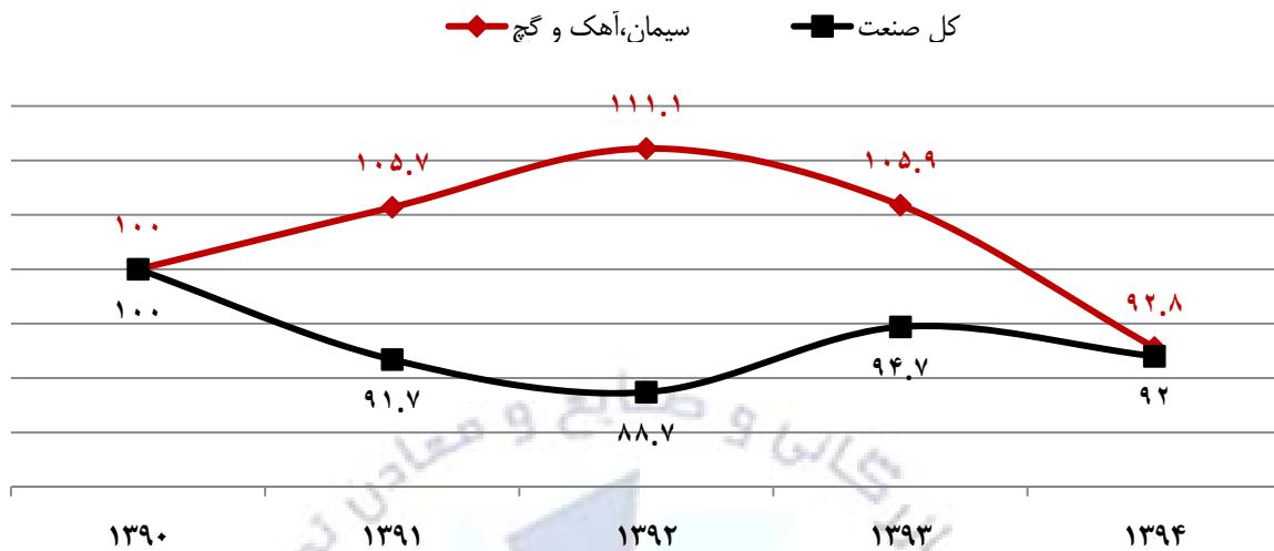
نمودار ۲ - روند سالانه شاخص تولید فعالیت سیمان، آهک و گچ و کل صنایع ۹۴-۱۳۹۰.
