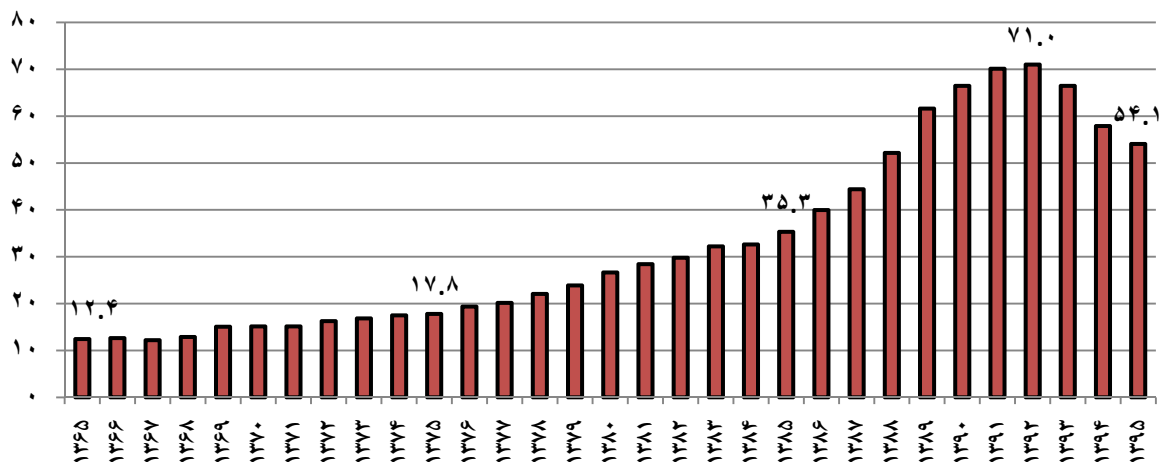
نمودار ۳ - روند سالانه میزان تولید سیمان در کشور ۹۵-۱۳۶۵، میلیون تن
