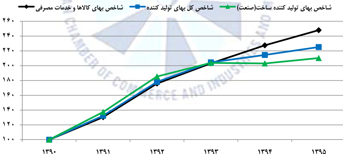
نمودار ۱- روند تغییر CPI، PPI و PPIM در سالهای ۱۳۹۰-۹۵ (۱۳۹۰=۱۰۰)
